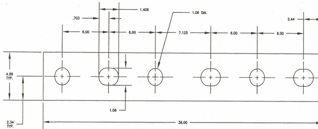
6 hole bar
